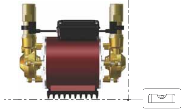
Şekil 5 Pompanın yerleştirilmesi
