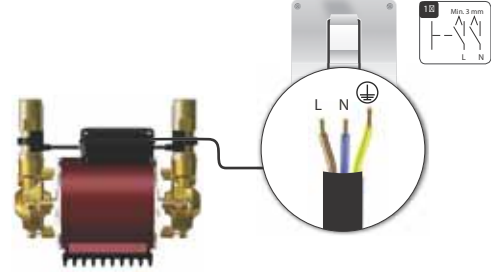
Şekil 23 Elektrik bağlantısı
