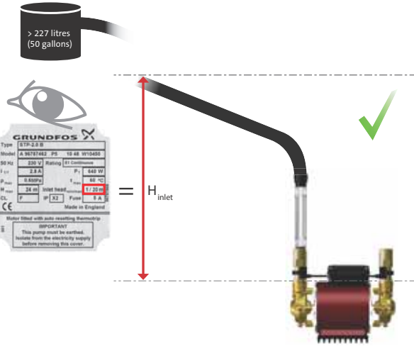
Şekil 3 Giriş basma yüksekliği
