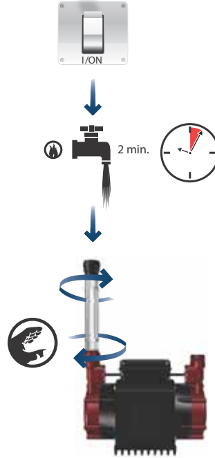
Şekil 29 Çalıştırdıktan sonra bağlantı yerlerini yeniden sıkın
